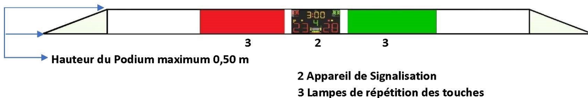
Figure 2 - PISTES NORMALES AUX TROIS ARMES
